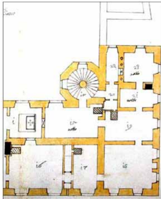
Die rechte Ecke des 1. Stockes nach dem Umbauplan der Grafen Lodron um 1654
