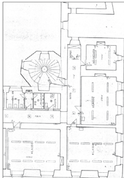
Die rechte Ecke des 1. Stockes nach dem Umbauplan des Schulgemeindevorstandes 1978
